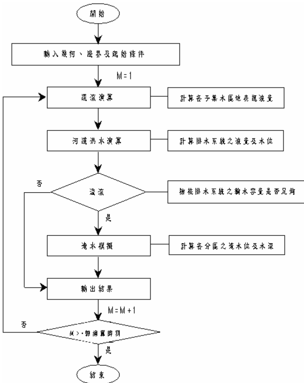
圖 3-2 淹水分析之演算流程圖
