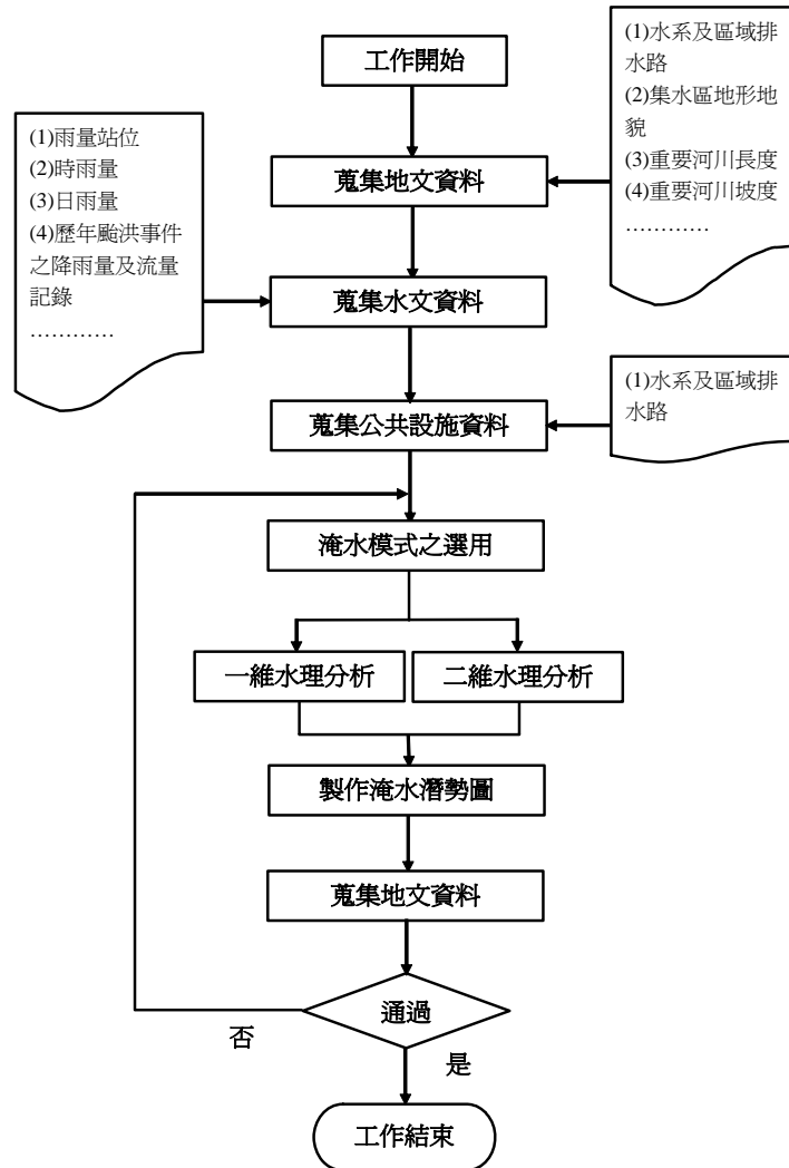
圖 2-1 淹水潛勢圖製作流程示意圖
